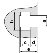
T groove dimensions (mm)
